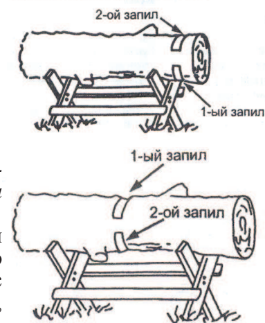
Использование стоящей опоры
